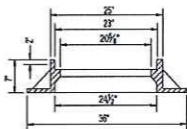
FRAME - TYPE I
